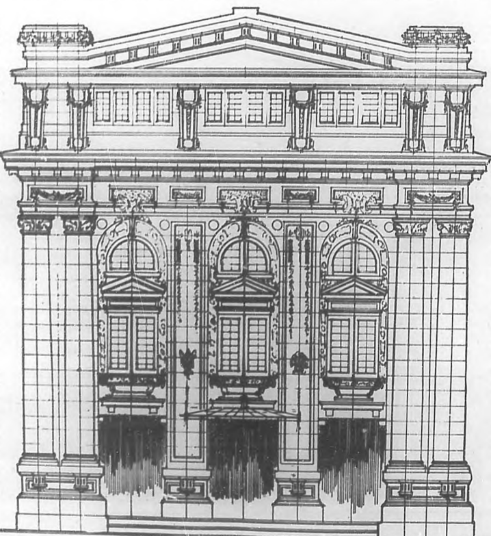
Proyecto de la fachada del hermoso edificio que se construirá para el "Teatro de la Comedia", en la calle de Consulado, en esta ciudad.
